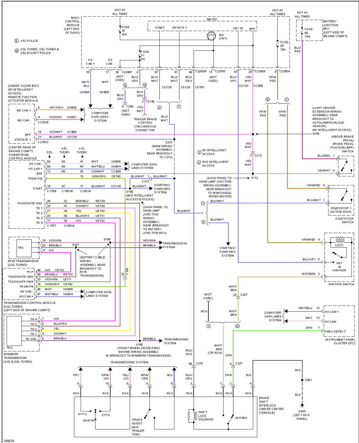
Fig. 114: Shift Interlock Circuit, W/ Floor Shift
