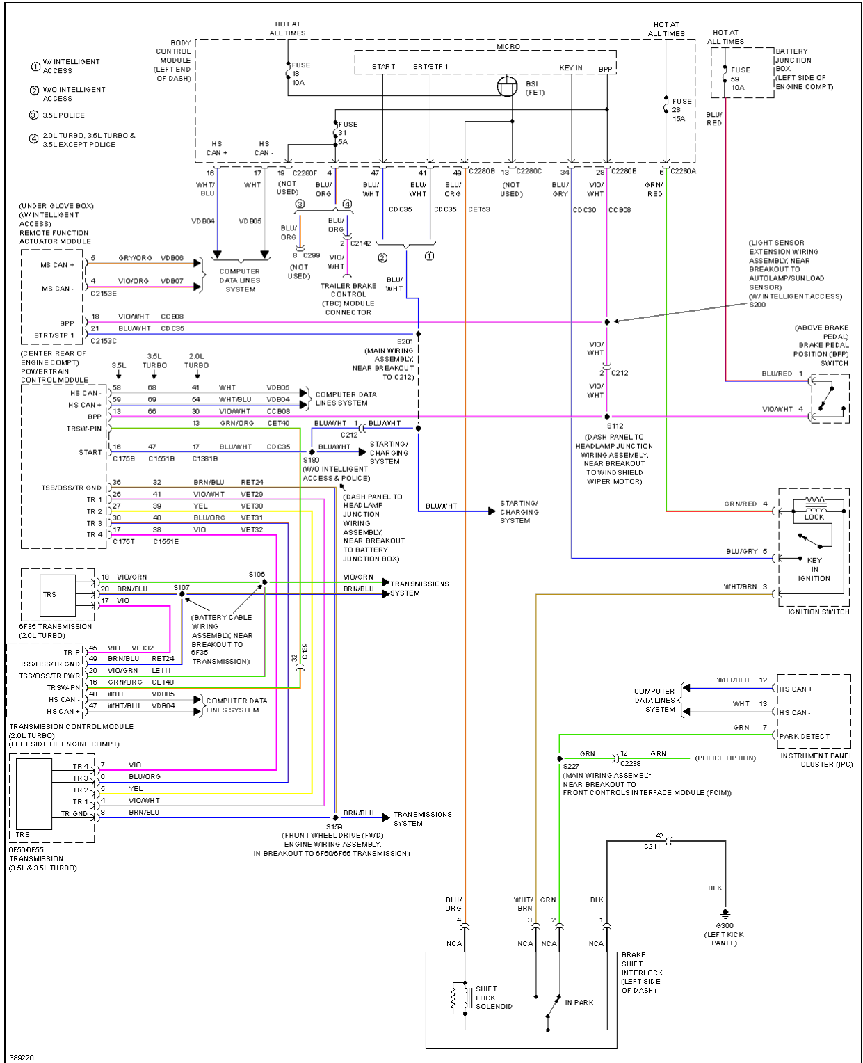
Fig. 113: Shift Interlock Circuit, W/ Column Shift
